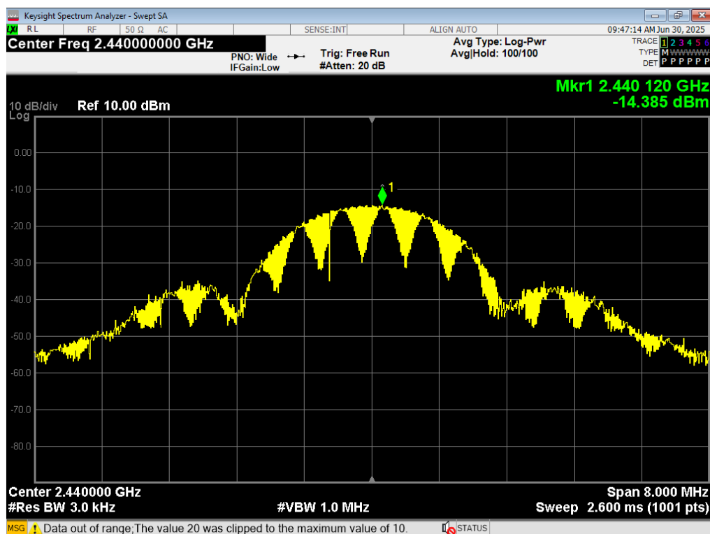
38 PSD, BLE 2MB, 2440MHz
