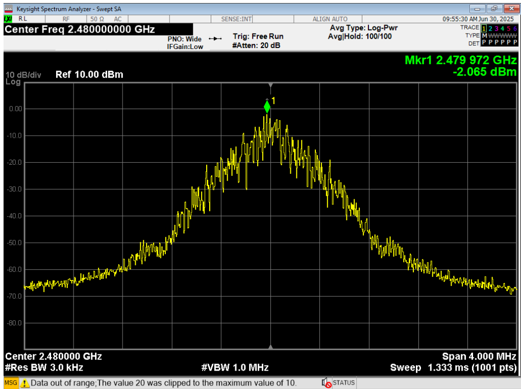
13 PSD, BTBR, 2480MHz
