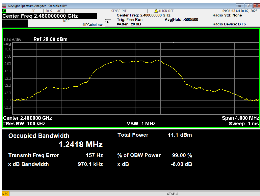
16 6dB BW, 3EDR, 2480MHz
