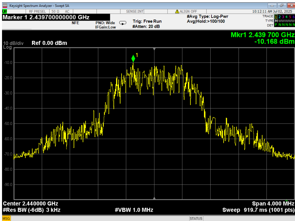
25 PSD, 3EDR, 2440MHz
