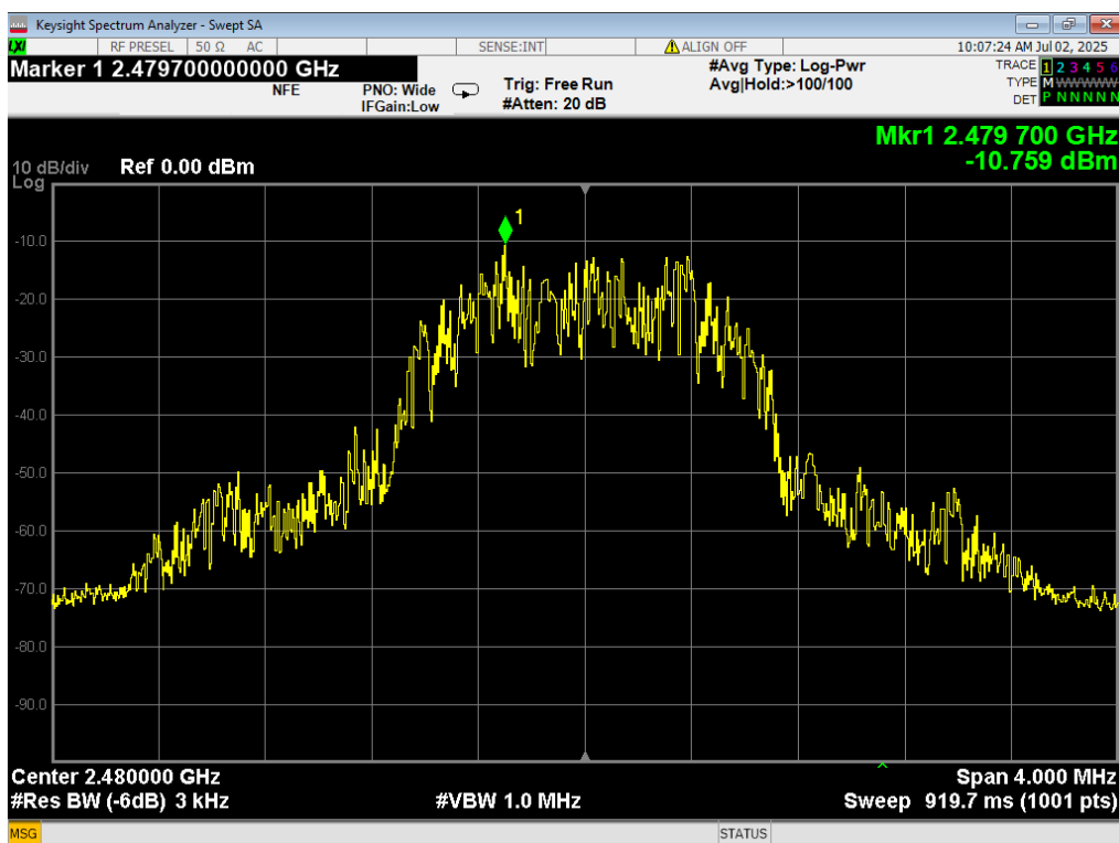
26 PSD, 3EDR, 2480MHz
