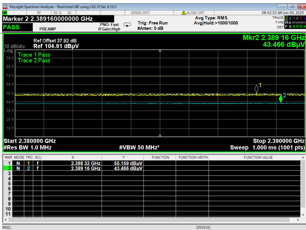
06 LBE Restricted, 2EDR, 2402MHz
