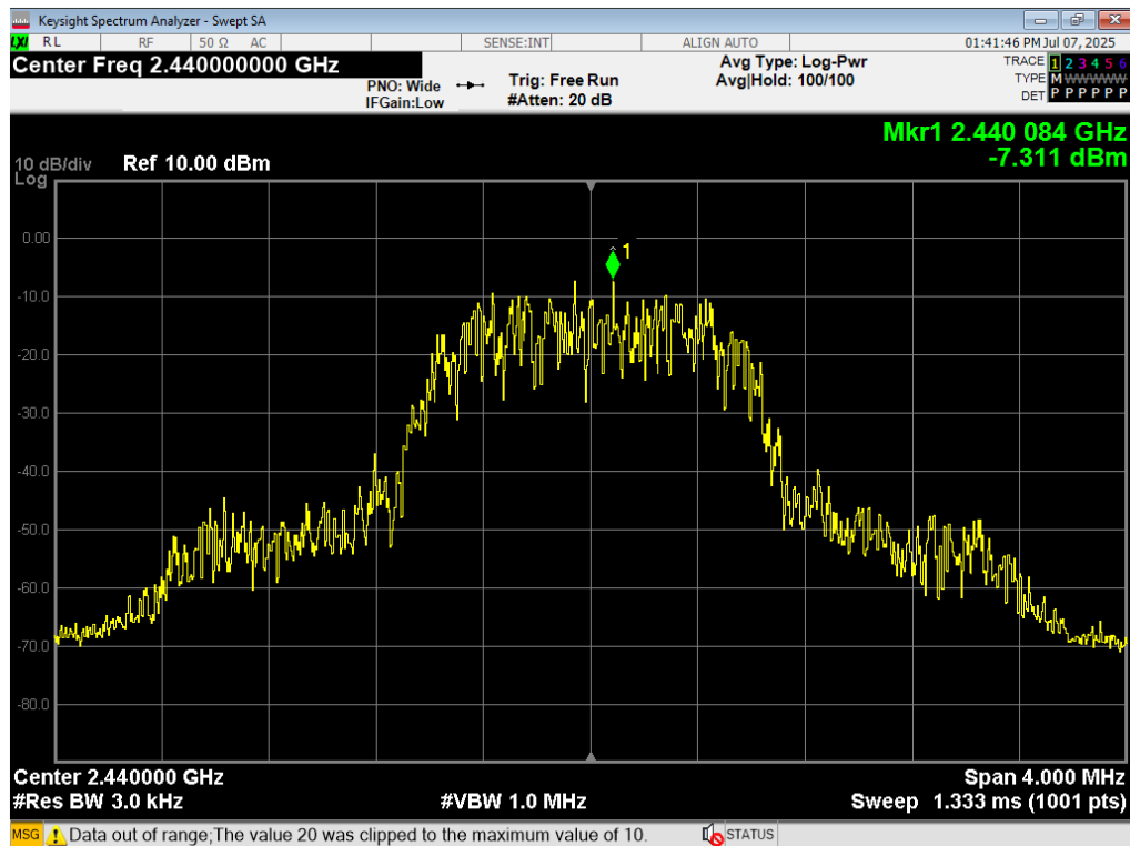
12 PSD, 2EDR, 2440MHz
