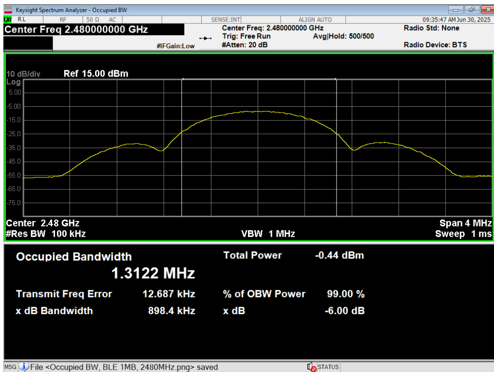
16 6dB BW, BLE 1MB, 2480MHz
