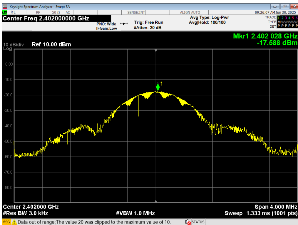
24 PSD, BLE 1MB, 2402MHz
