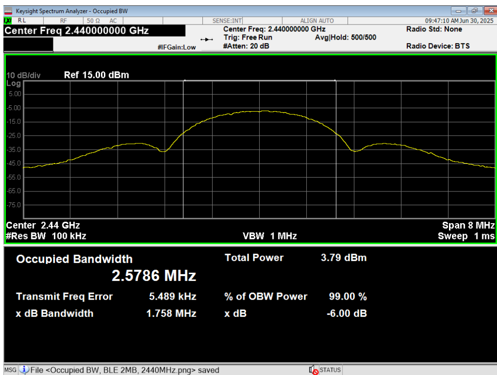
28 6dB BW, BLE 2MB, 2440MHz
