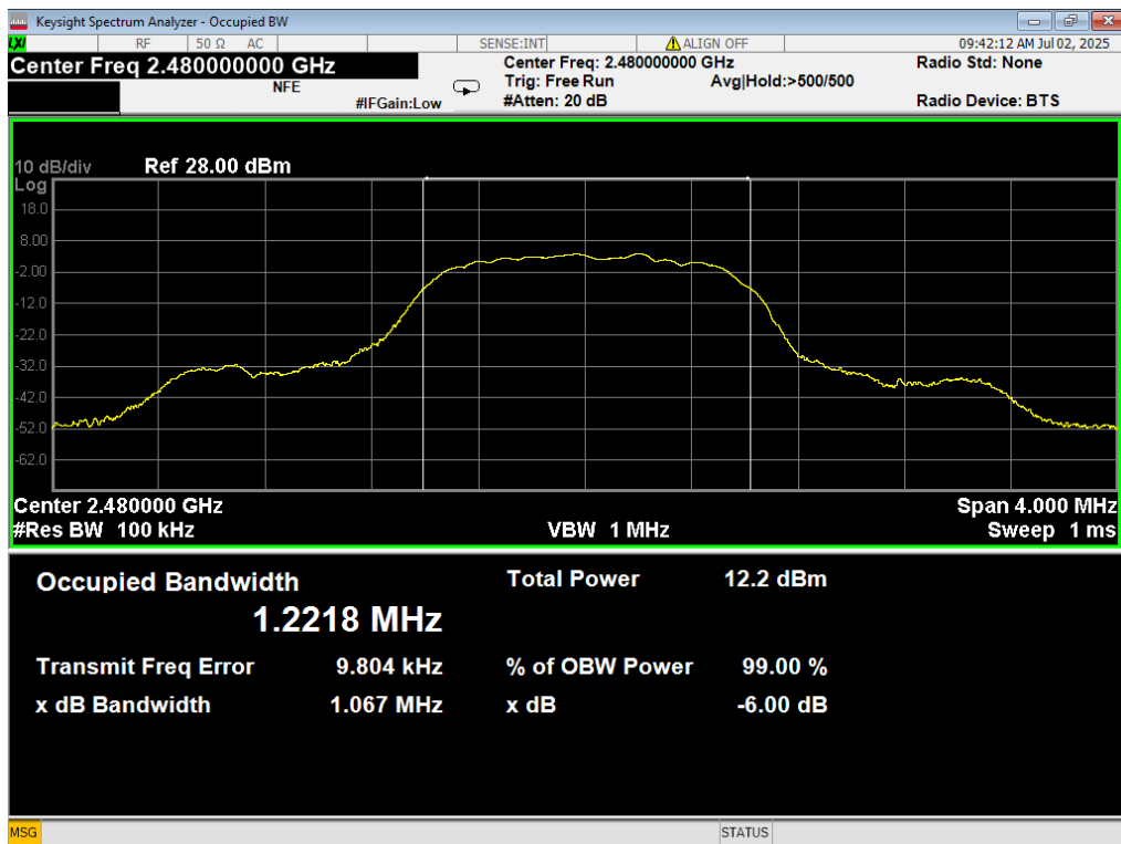
03 6dB BW, 2EDR, 2480MHz
