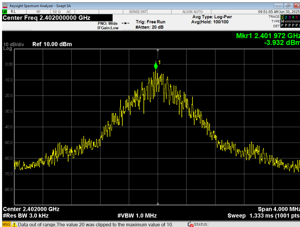
11 PSD, BTBR, 2402MHz
