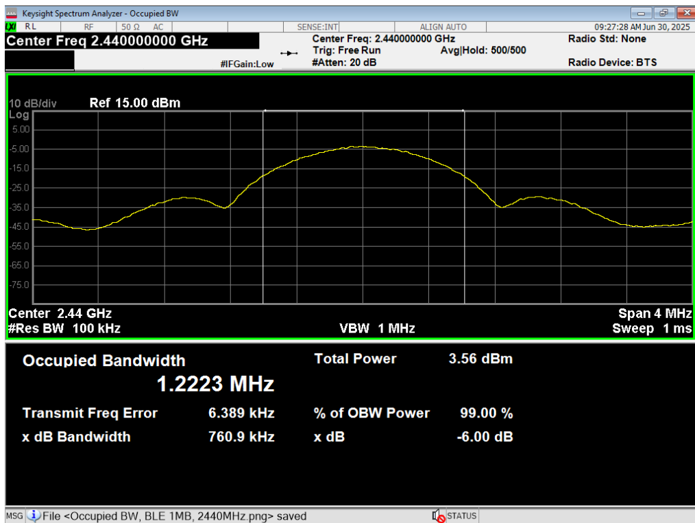
15 6dB BW, BLE 1MB, 2440MHz
