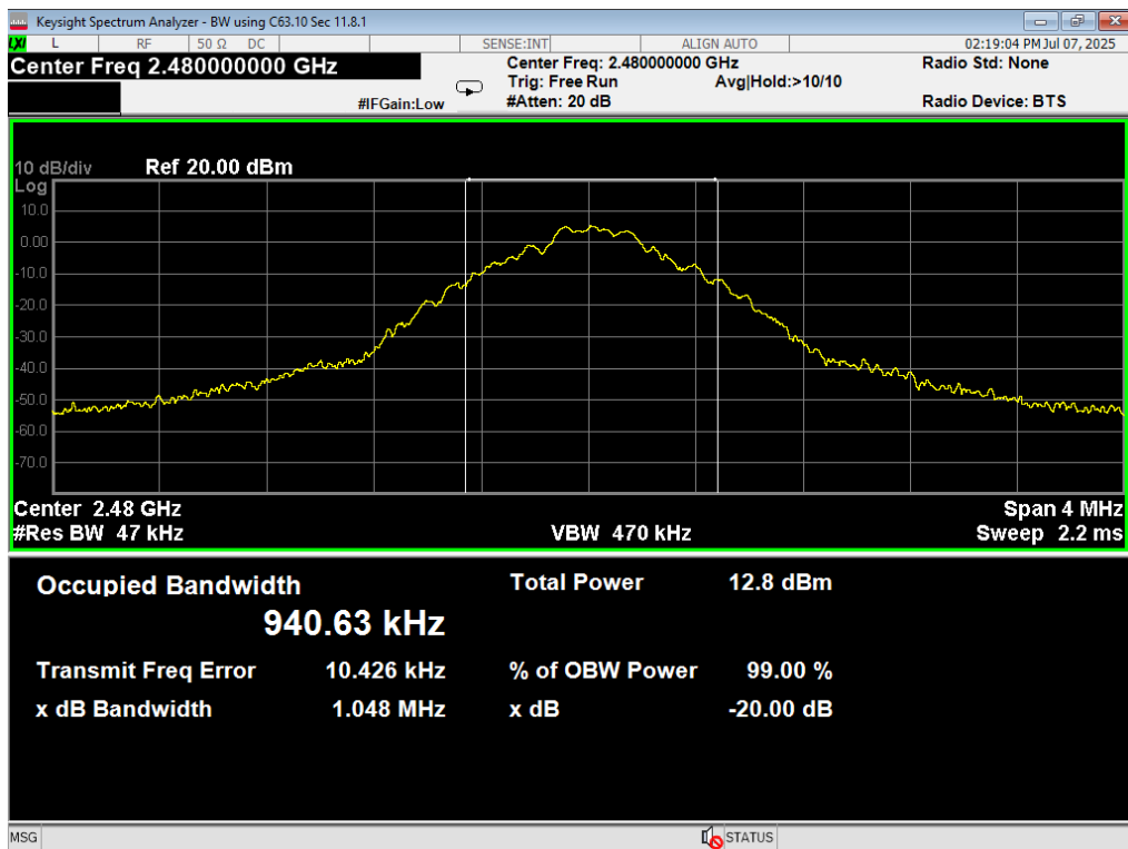
03 20dB BW, BTBR, 2480MHz
