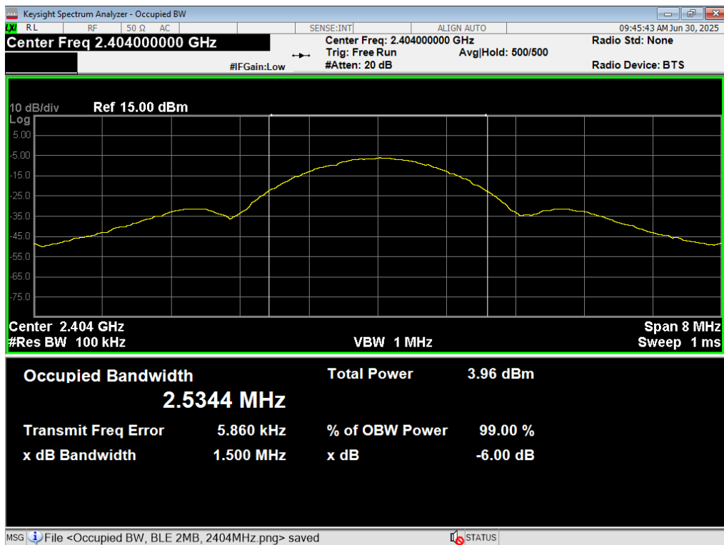
27 6dB BW, BLE 2MB, 2404MHz
