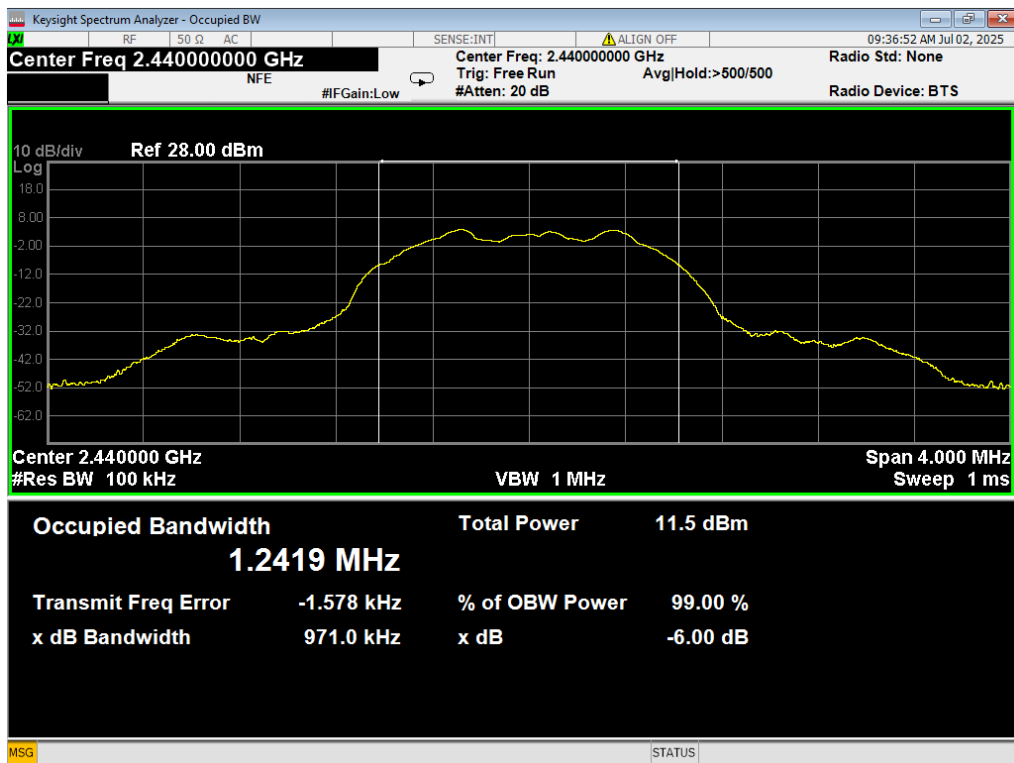
15 6dB BW, 3EDR, 2440MHz
