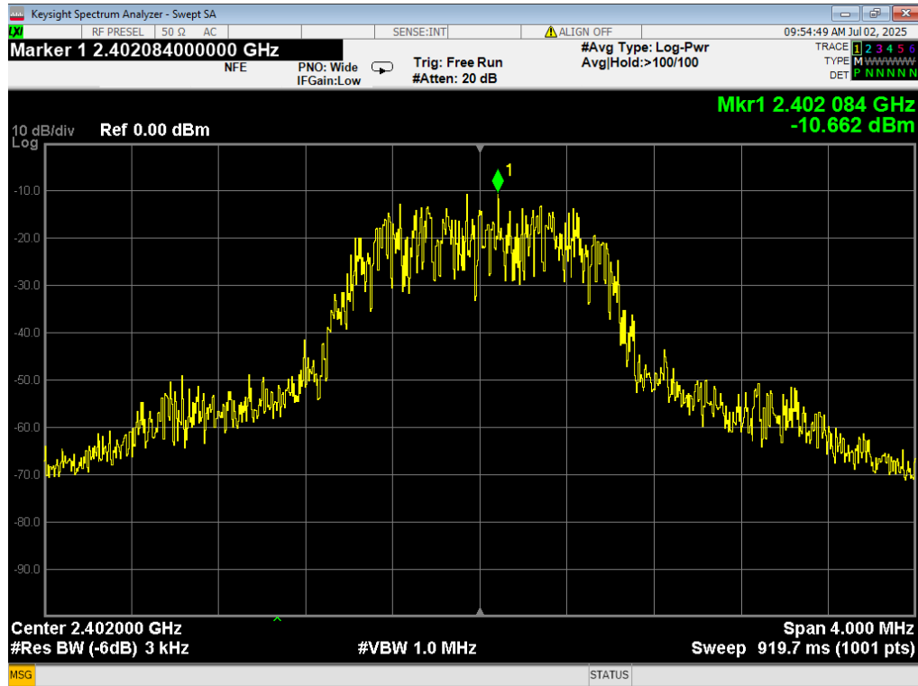
11 PSD, 2EDR, 2402MHz
