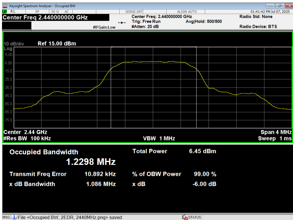
02 6dB BW, 2EDR, 2440MHz
