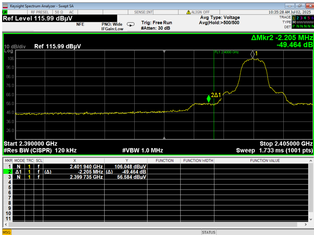
07 LBE Unrestricted, 2EDR
