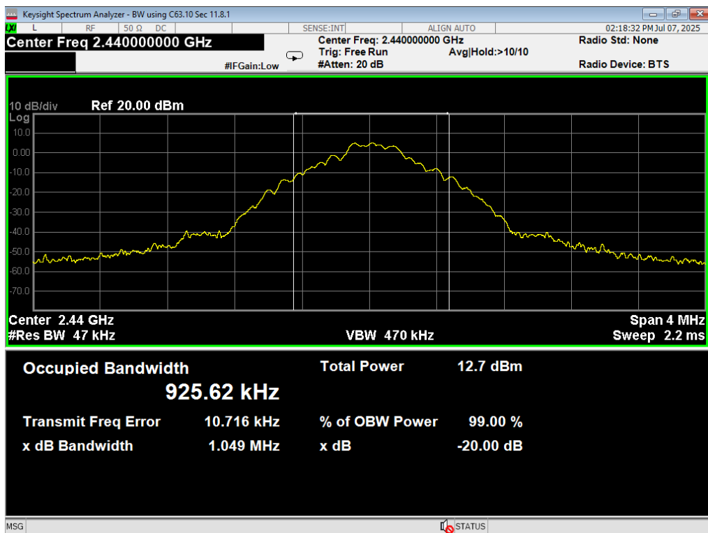
02 20dB BW, BTBR, 2440MHz
