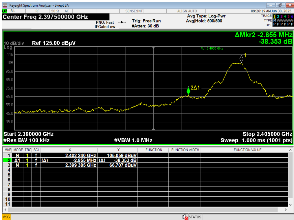
20 LBE Unrestricted, BLE 1MB, 2402MHz
