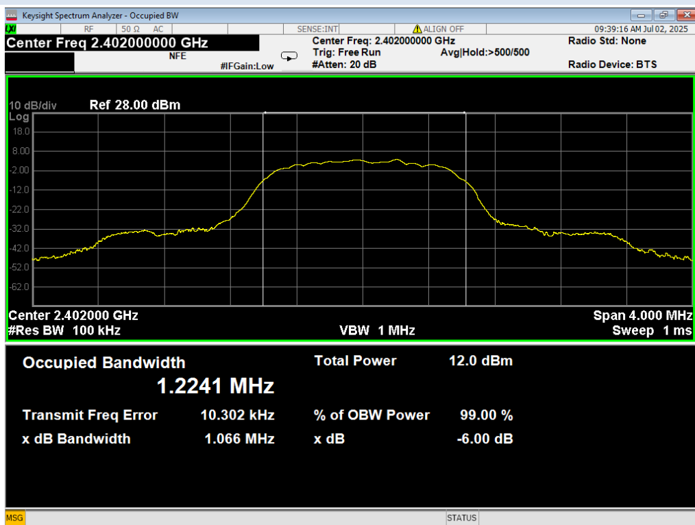
01 6dB BW, 2EDR, 2402MHz
