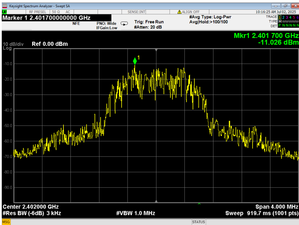
24 PSD, 3EDR, 2402MHz
