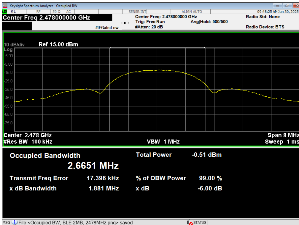
29 6dB BW, BLE 2MB, 2478MHz
