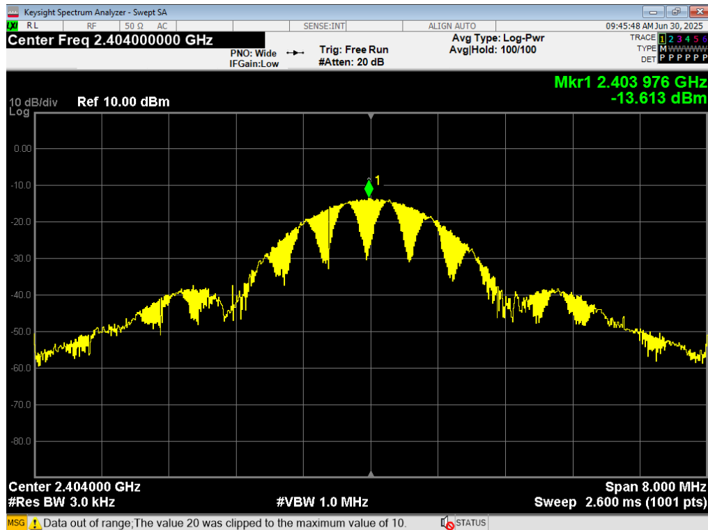
37 PSD, BLE 2MB, 2404MHz
