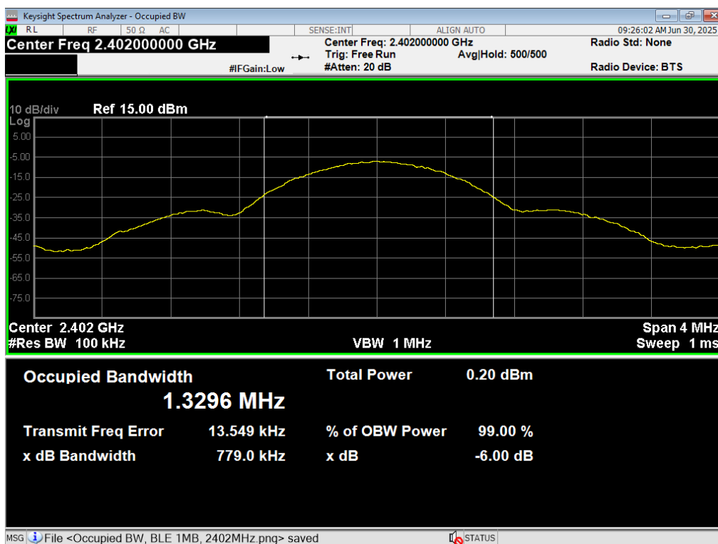
14 6dB BW, BLE 1MB, 2402MHz
