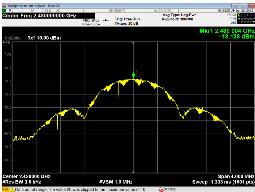
26 PSD, BLE 1MB, 2480MHz
