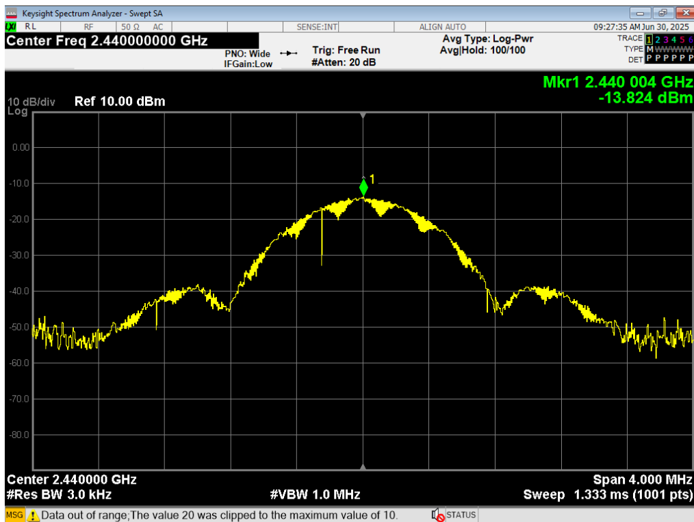
25 PSD, BLE 1MB, 2440MHz
