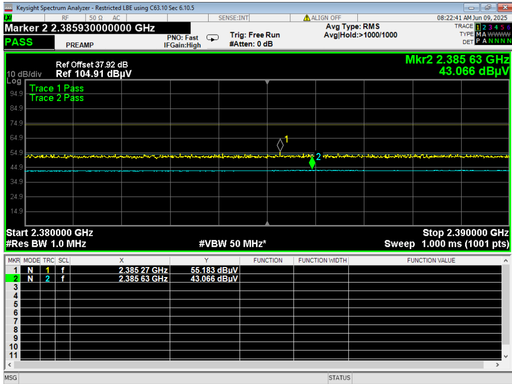
19 LBE Restricted, BLE 1MB, 2402MHz
