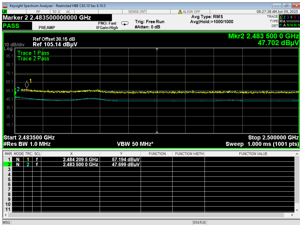
17 HBE Restricted, BLE 1MB, 2480MHz
