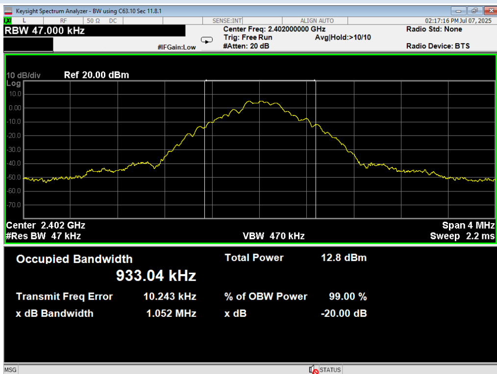
01 20dB BW, BTBR, 2402MHz
