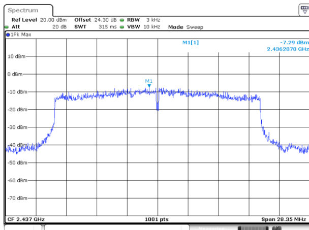
MIMO Ant. 6
