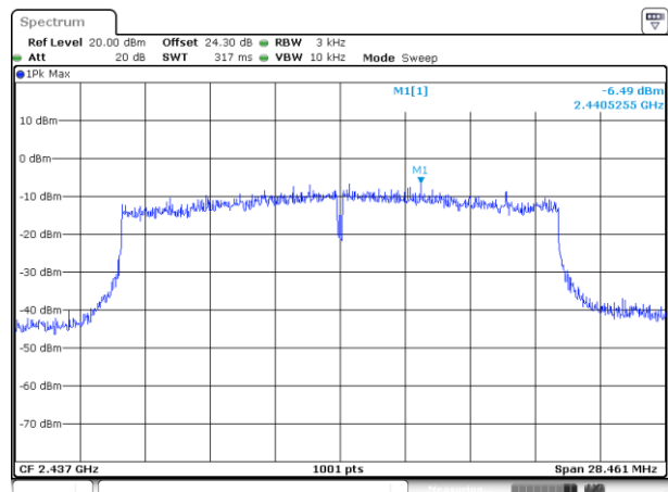
MIMO Ant. 7
