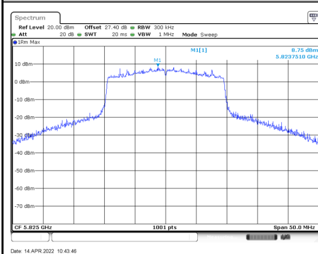
MIMO Ant. 6
