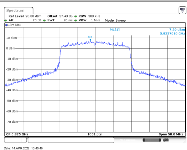
MIMO Ant. 7
