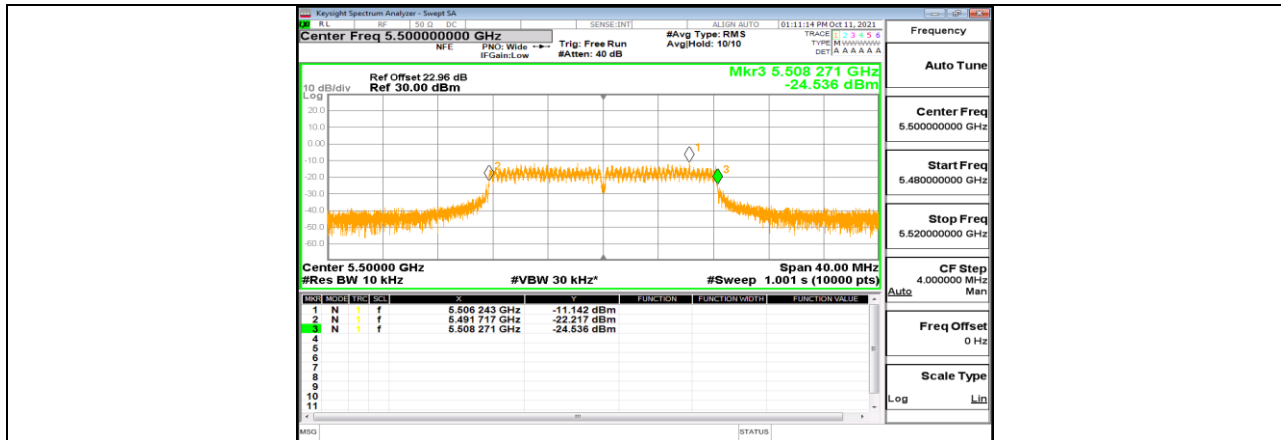
HTNV 11A Ant1 5500
