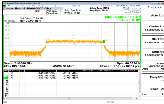
NTNV 11N20MIMO Ant2 5500
