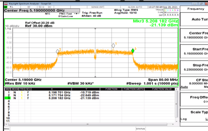
NTNV 11N40MIMO Ant2 5190
