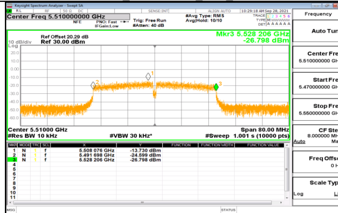
NTNV 11N40MIMO Ant2 5510
