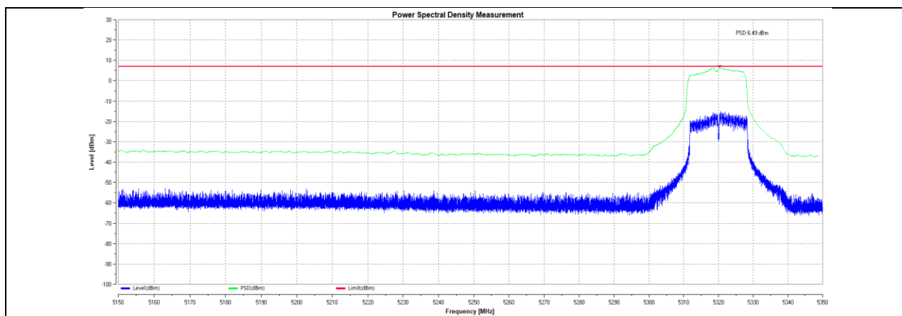
11A_Ant2_5320
