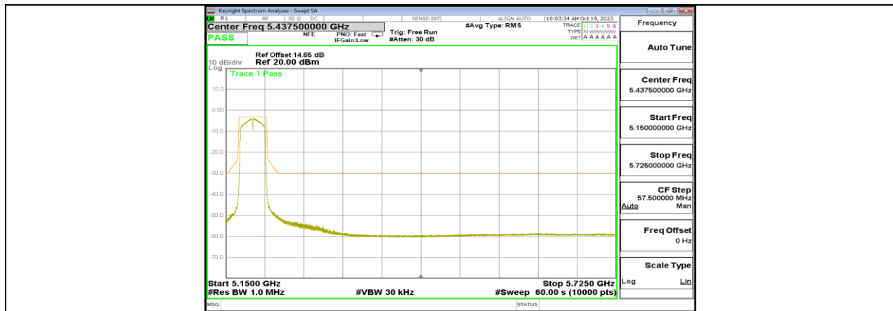
11N40MIMO Ant1 5190
