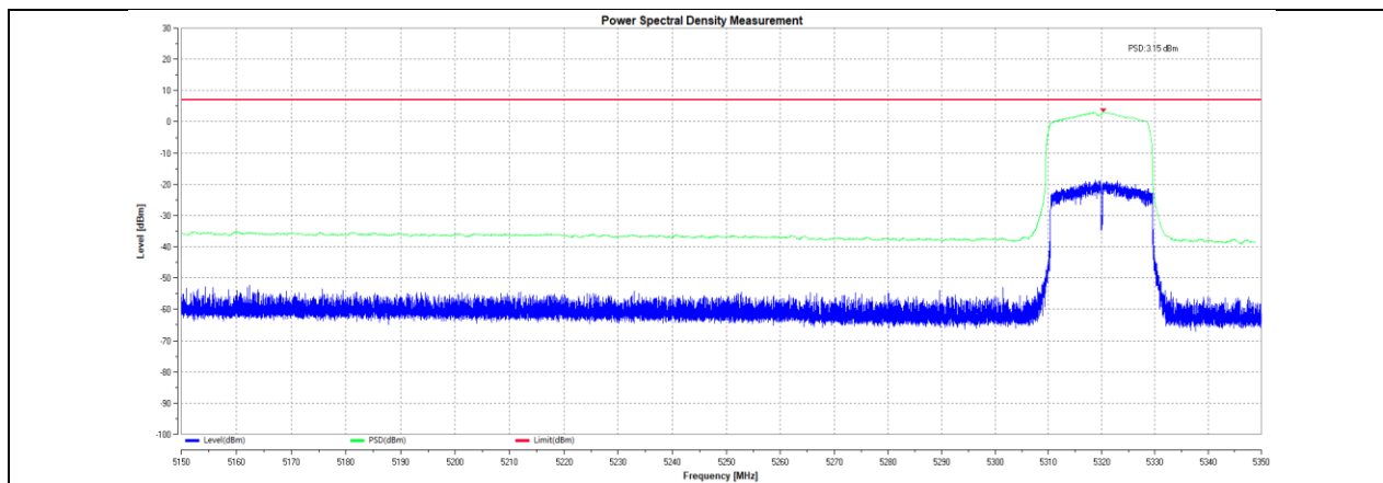
11AX20MIMO_Ant2_5320
