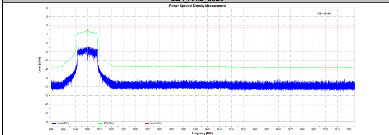
11A_Ant1_5500
