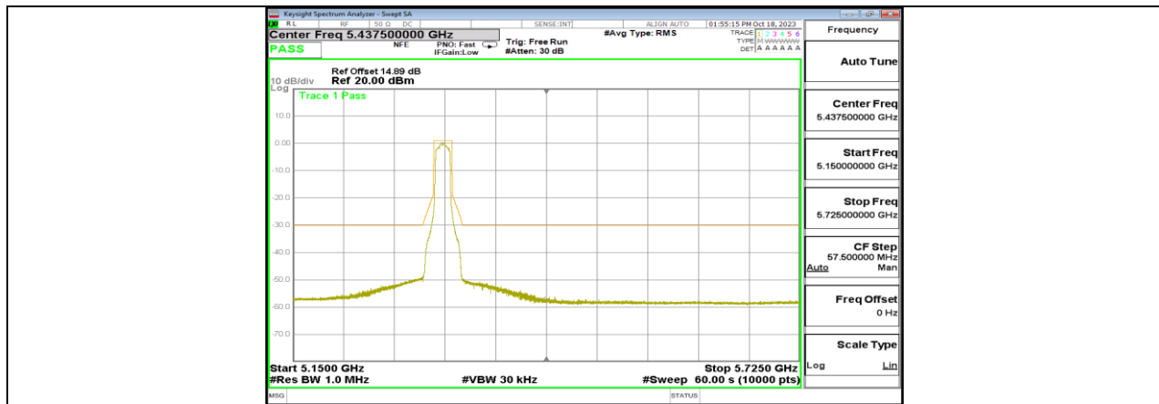
11A Ant1 5320
