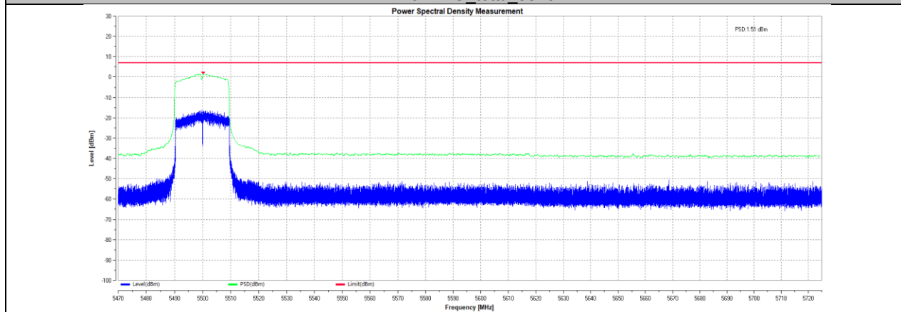
11AX20MIMO_Ant1_5500
