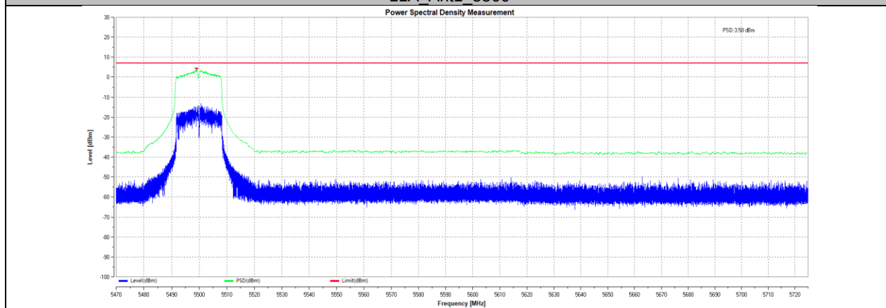
11A_Ant2_5500
