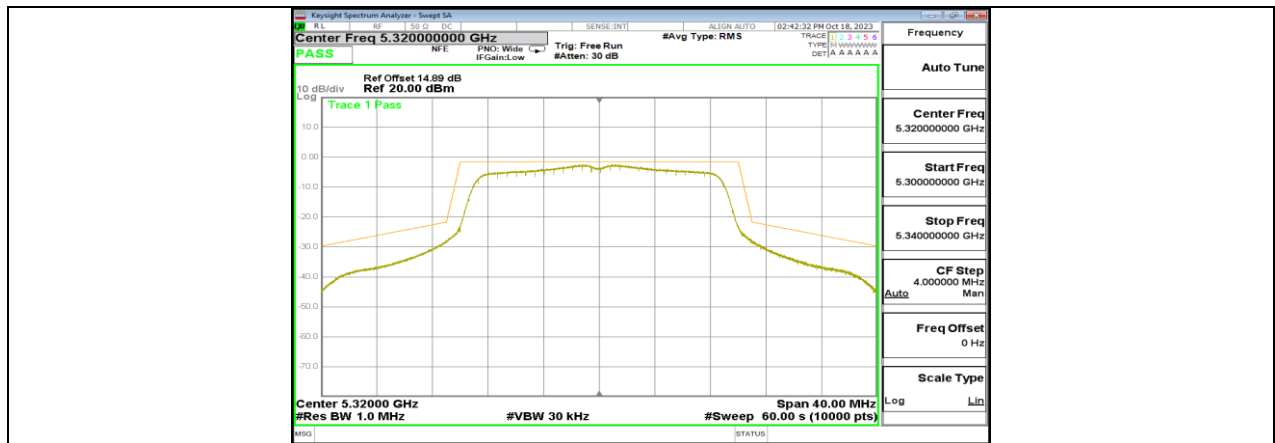
11N20MIMO Ant1 5320
