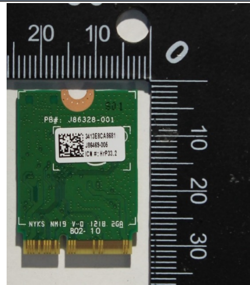
Module Back
